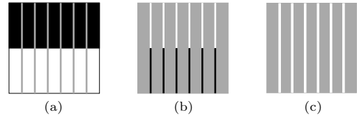
図 7 遮へい領域と背景領域のコントラストの関係が変化する場合 (a) 画像例。細い灰色の領域が遮へい領域である。(b) 投票量の分布。白色、灰色、黒色はそれぞれ正、0、負の投票量を表す。(c) 符号判別後の投票量の符号。白色と灰色は、それぞれ正と 0 の投票量を表す。
