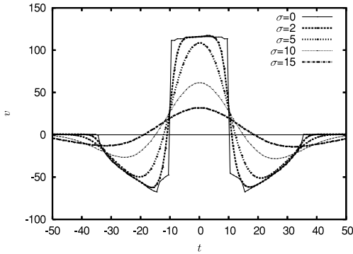
図 6 画像が標準偏差 \sigma のガウス関数でぼかされたときの投票量 v の距離 t に対するプロット ( w = 20, a = 255, b = 0, r_1 = 25 )
