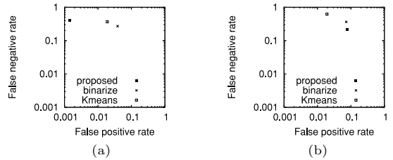
図 20 本手法と 2 値化, 領域分割の定量的な比較 (a) 図 19 (a) の抽出結果 (b) 図 19 (d) の抽出結果 Fig. 20 Quantitative comparison with binarization and segmentation (a) result of Fig. 19 (a). (b) result of Fig. 19 (d).
