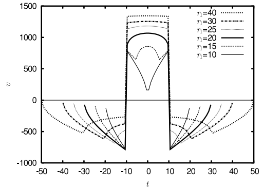
図 5 半径 r_1 を変化させたときの投票量 v の距離 t に対するプロット ( w = 20, a = 255, b = 0 )
