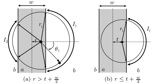
図 3 注目画素が遮へい領域上に存在する場合 ( t < \frac{w}{2} ) の投票モデル
