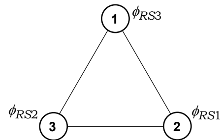
図12. 操作 RS を施された基底
