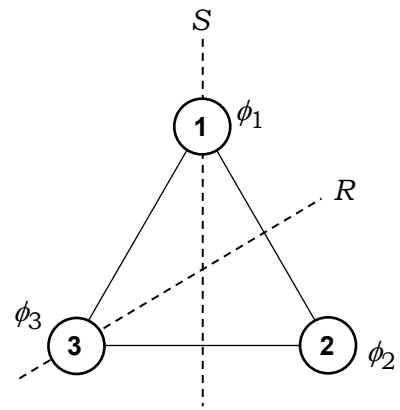
図6. 正三角形形状分子の基底
