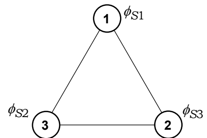
図10. 操作 S を施された基底
