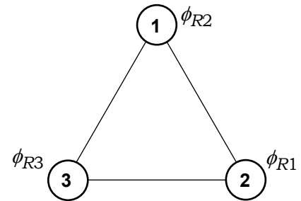
図11. 操作 R を施された基底
