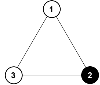
図8. 操作 R を施した結果 R\psi
