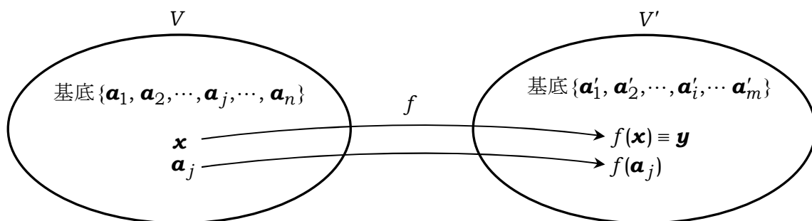
図13. 空間 V から空間 V' への1次写像
