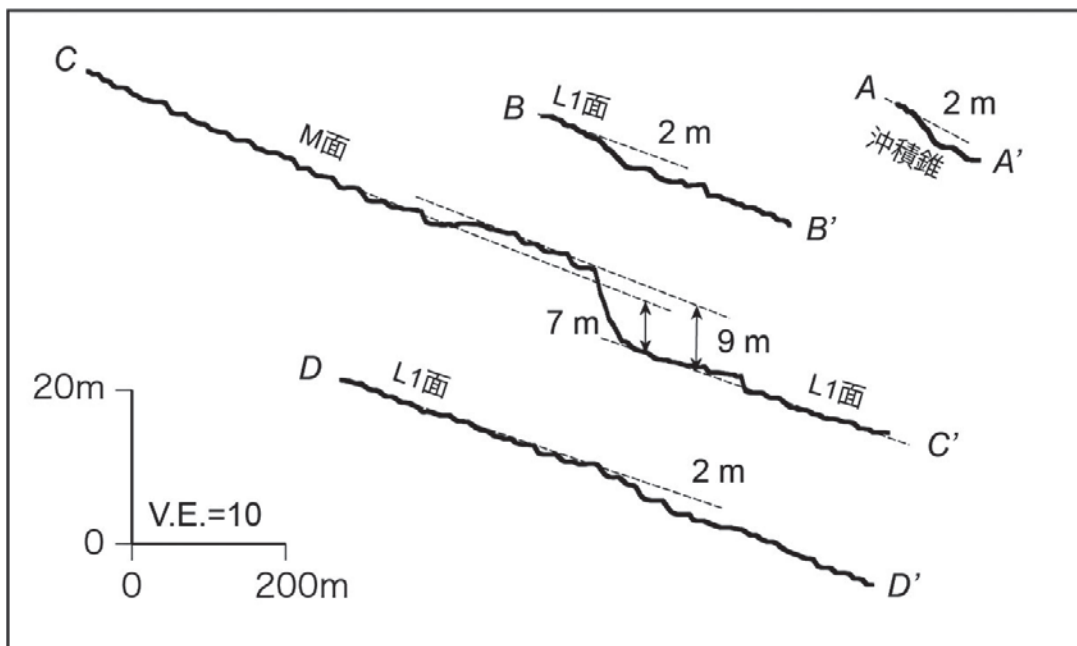
図4 地形断面図
