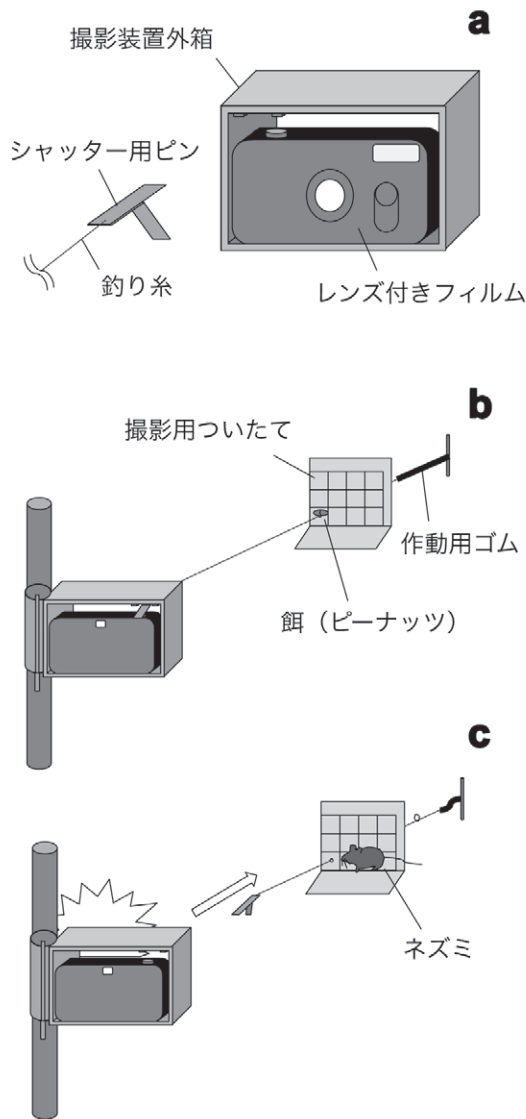
図 2. ネズミ類用の自動撮影装置
