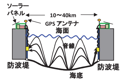
沿岸音響トモグラフィー装置
