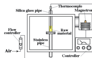
粉体流動型マイクロ波加熱反応装置概略
