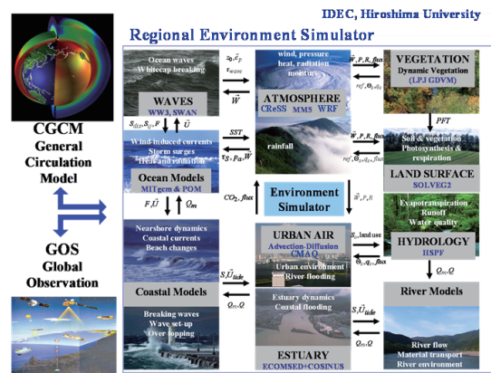
地域環境シミュレーター (RES)
