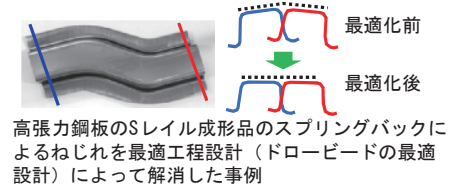
高張力鋼板のSレール成形品のスプリングバックによるねじれを最適工程設計（ドローベンドの最適設計）によって解消した事例
