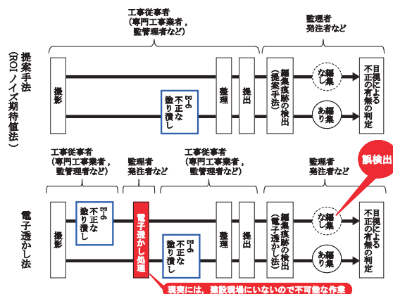
図2 提案手法の優位性 工事の従事者による前処理作業が不要
