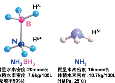
図 1. アンモニアボランとアンモニアの構造
