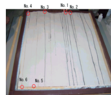
原爆資料館「黒い雨」壁面とガンマ線スペクトル
