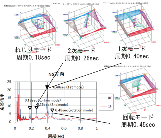
図2 応答倍率 (フーリエスペクトル比)
