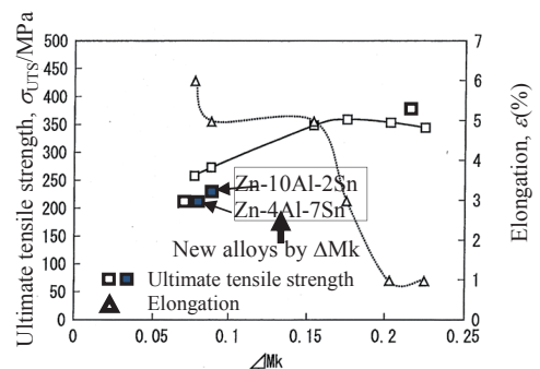
図 1 \Delta Mk と強度, 伸びの関係
