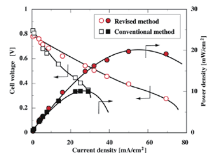
焼却飛灰を再資源化したゲル膜を持つ燃料電池の発電特性
