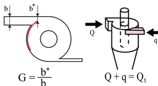
開発した高性能サイクロン
