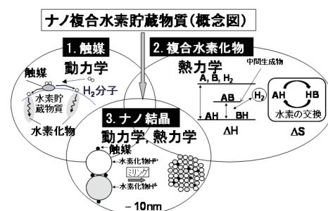
図 2. ナノ複合水素貯蔵物質の概念図 (ΔH: エンタルピー差, ΔS: エントロピー差, AH, BH: 水素化物, 水素化物のサイズ: 10-100nm)
