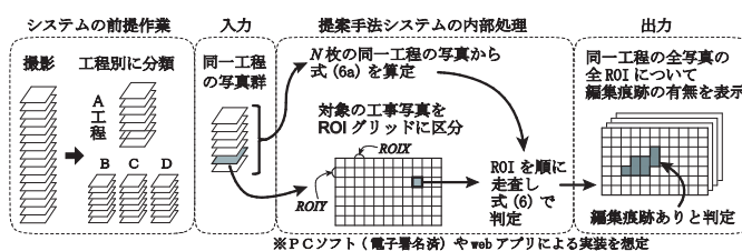
図1 システムの概要図
