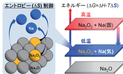
非平衡プロセスによる反応温度制御の概念図
