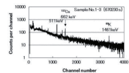
原爆資料館「黒い雨」壁面とガンマ線スペクトル
