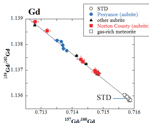
同位体比の変動を示す Gd の 3 同位体プロット。標準値 (STD) に対して宇宙線照射の影響を受けた隕石試料の Gd 同位体比が顕著にが変動している。
