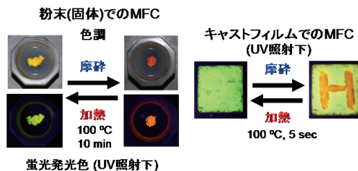
D- \pi -A 型蛍光性色素 1a-5a
